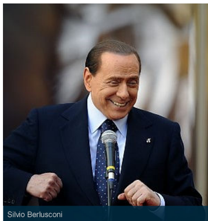
Silvio Berlusconi
